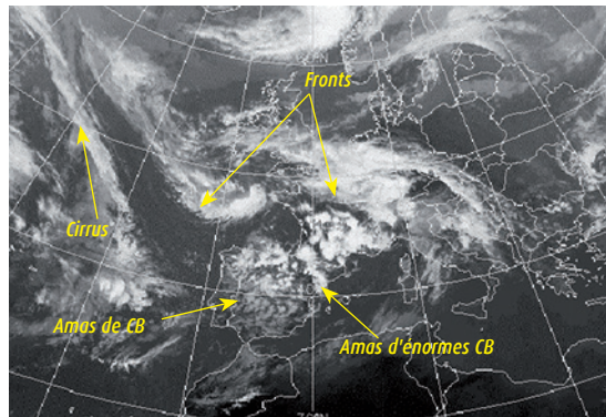
Image infrarouge sur l'Europe
